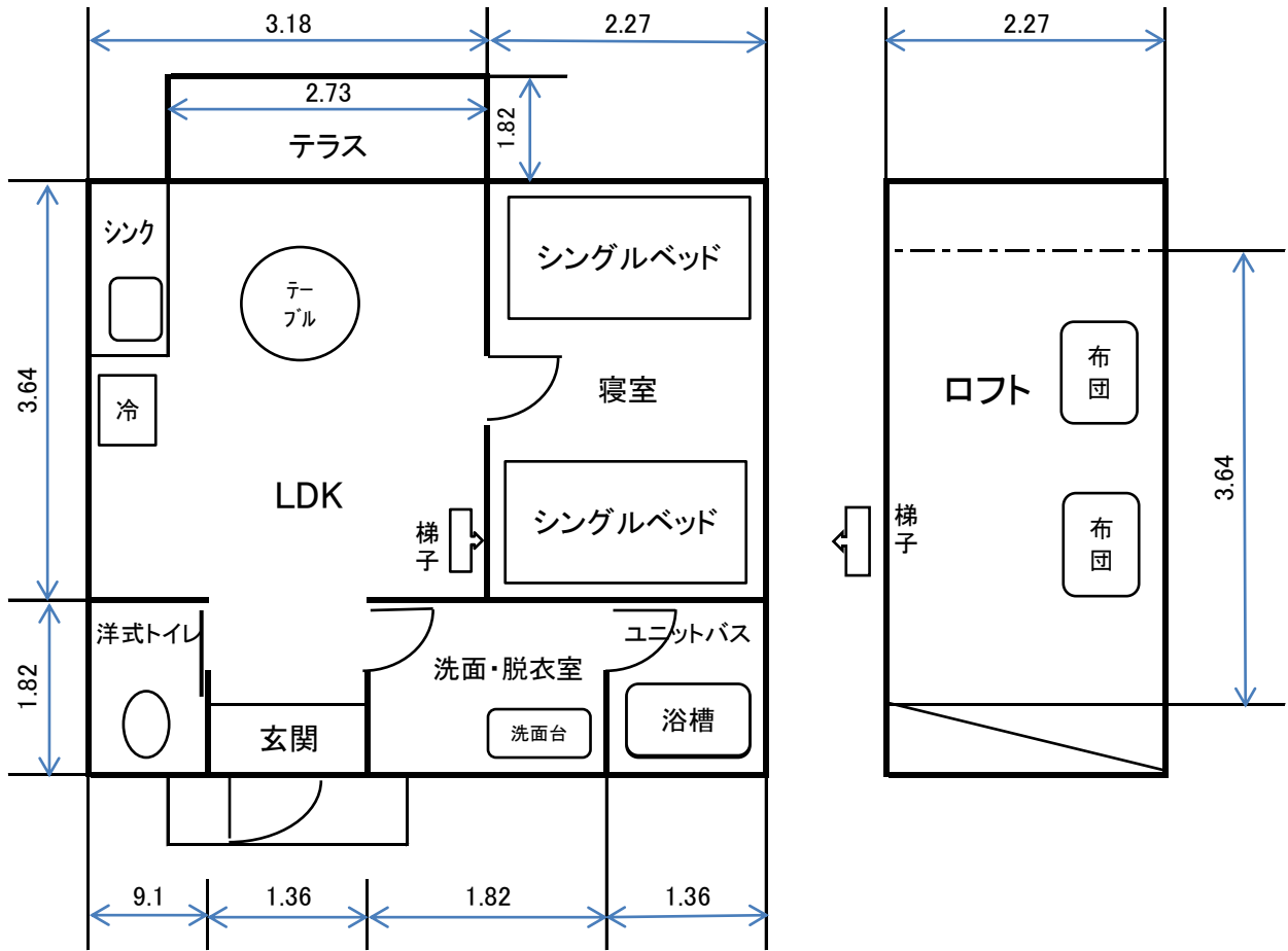
コテージA(定員5人タイプ)平面図(概略)
